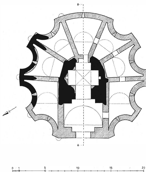
FIG. 8 - Torraccia dell'Inviolata: ipotesi ricostruttiva della pianta.
