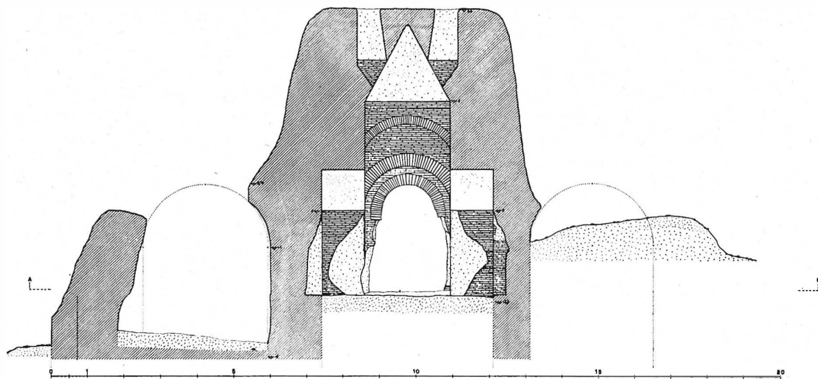
FIG. 9 - Torraccia dell'Inviolata: sezione.
