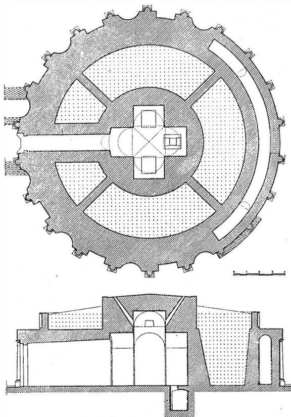
FIG. 19 - S. MARIA CAPUA VETERE, Carceri Vecchie: pianta e sezione.
