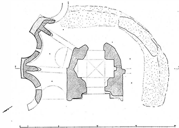
FIG. 4 - Torraccia dell'Inviolata: pianta.
