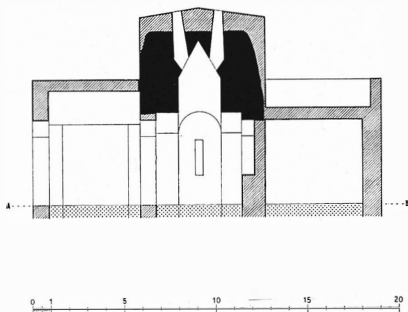
FIG. 16 - Torraccia dell'Inviolata: ipotesi ricostruttiva dell'alzato.
