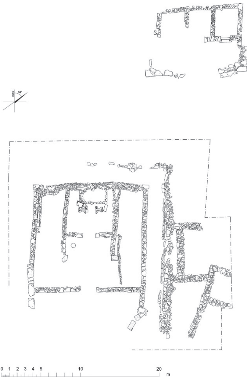
Fig. 2 Planimetria dell' Aerarium e di uno dei due thesauroi con tre ambienti affacciati su un porticato. – (Elaborazione grafica di S. Polvere, 2017).
